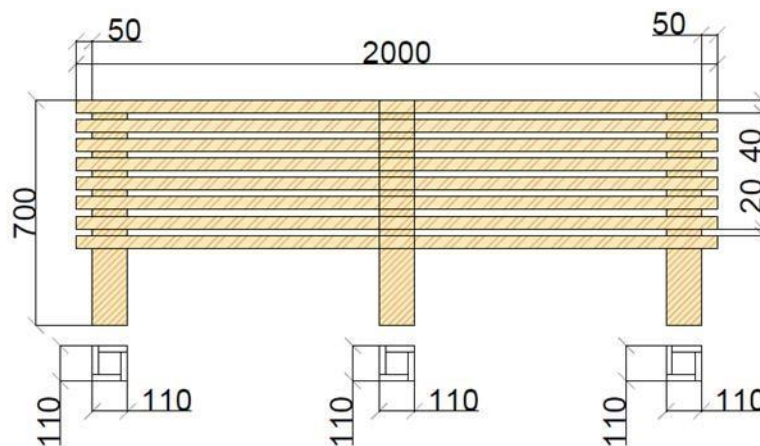
Рис. 2. Эскиз Забора
